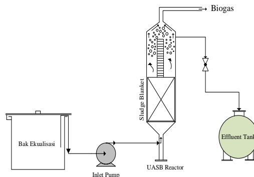
Gambar 3. Rancangan Reaktor UASB
