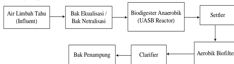
Gambar 2. Rancangan Instalasi Pengolahan Air Limbah (IPAL)
