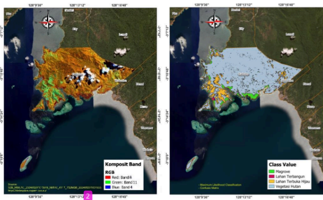
Gambar 2. Hasil Komposit Band (8 11 4) dan Hasil Klasifikasi
