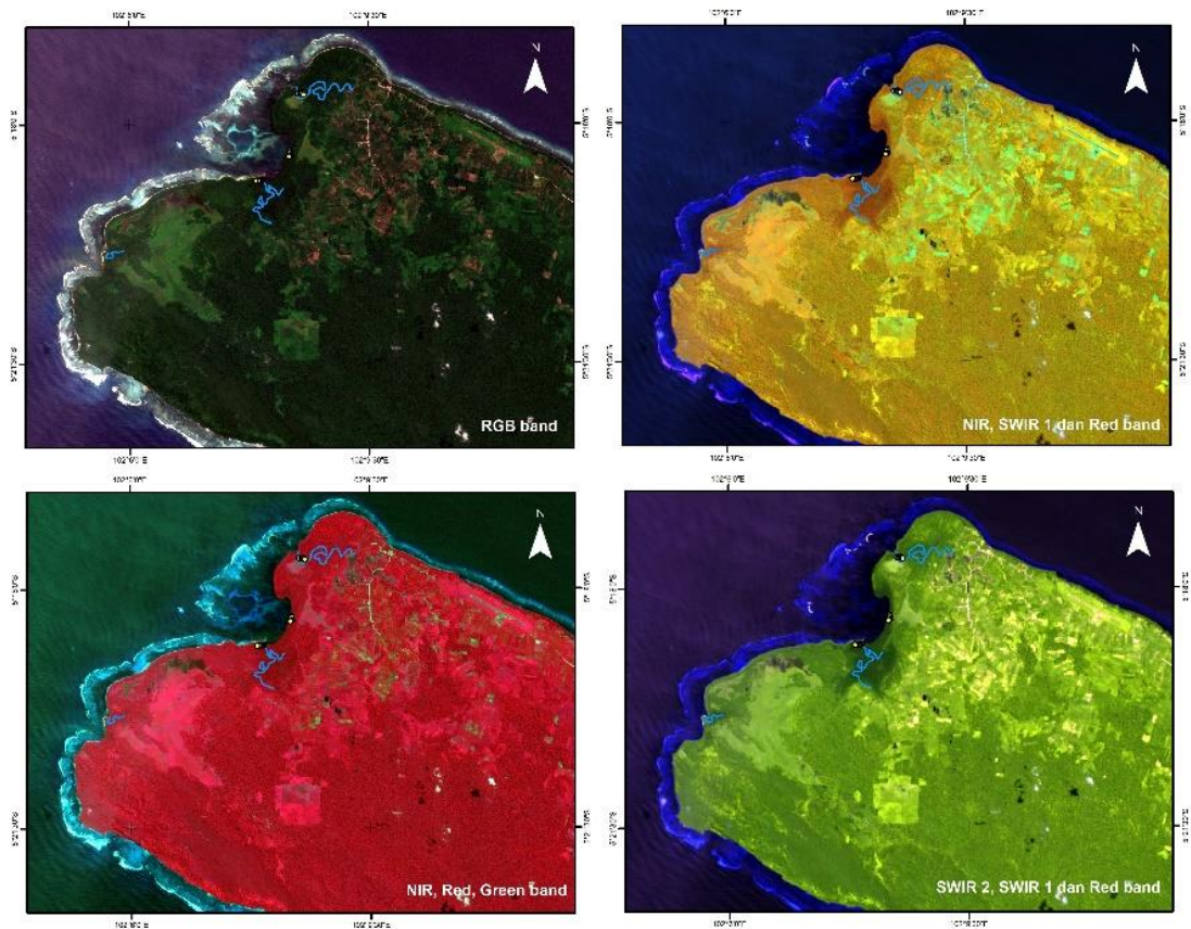
Gambar 2. Kombinasi false dan true color band Sentinel-2A
