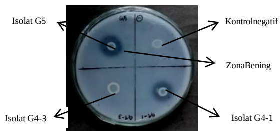
Gambar 2. Aktifitas pelarutan fosfat oleh bakteri sedimen gua
