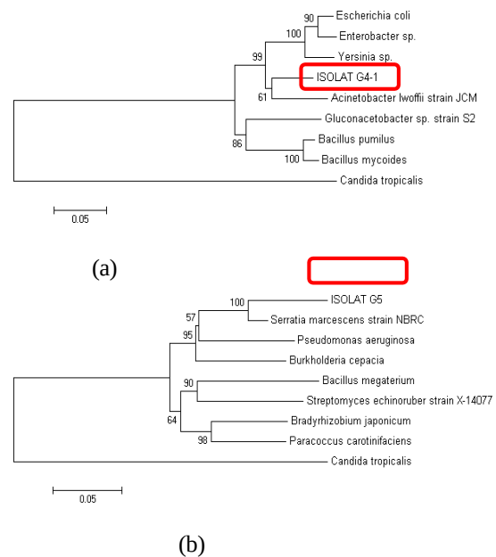
Gambar 5. Pohon Filogenetik 16s rRNA menunjukkan posisi sekuen isolat bakteri G4-1 dan G5 dengan sekuen homolog. Metode NJ digunakan untuk pembuatan pohon filogenetik dengan model perhitungan p-distance .
