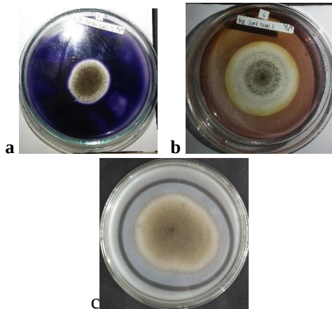
Gambar 1. Zona bening yang terbentuk (a) amilase (b) selulolulase (c) protease
